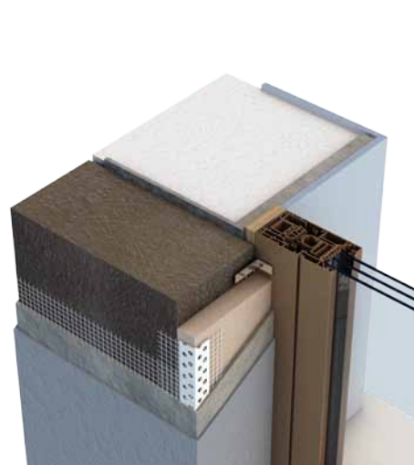
PUR - purenitové ostění
